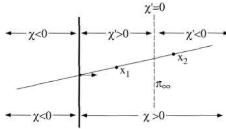
Fig. 21.5. The parameter \chi .
